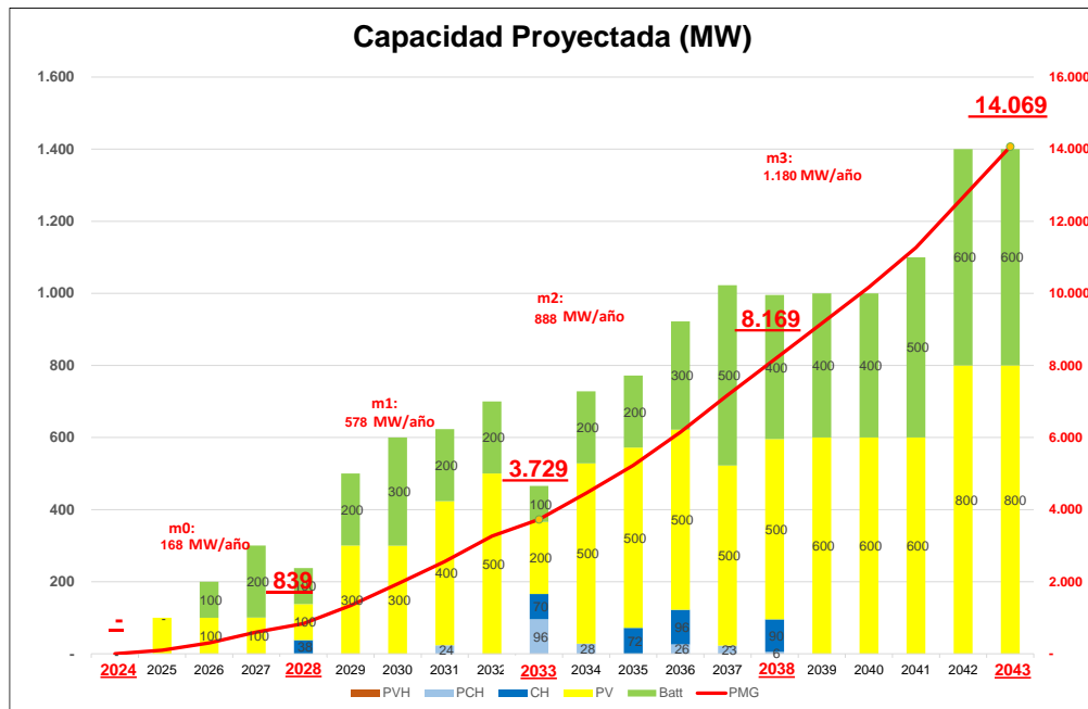
Fig. 4.1. Plan A. Evolución de la Capacidad de Generación 2024-2043
