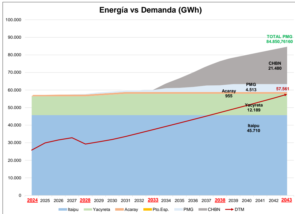
Fig. 4.7 Plan C/D. Evolución de la Producción de energía esperada 2024-2043.
