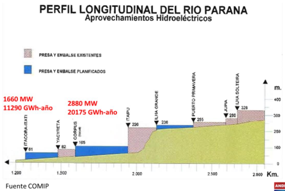
Fig. 3.1 – Perfil longitudinal del Río Paraná Central Hidroeléctrica de Itacorá-Itatí (CHBN-ItIt)
