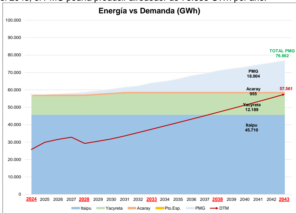
Fig. 4.6 Plan B. Evolución de la Producción de energía esperada 2024-2043.
