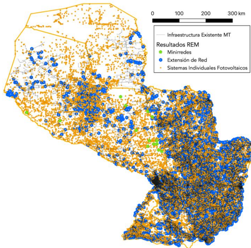
Fig. 5.2 Ubicación de las obras
