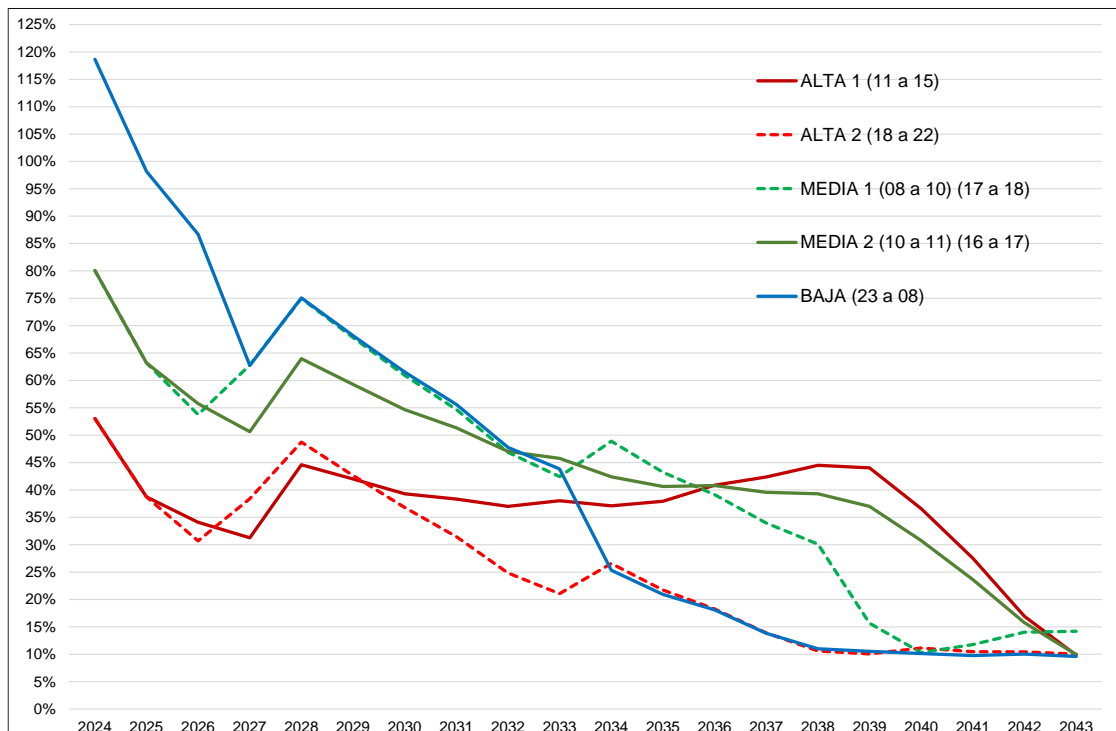
Fig. 4.9 Plan B. Evolución de los Márgenes de Reserva de Potencia (MRP) 2024-2043
