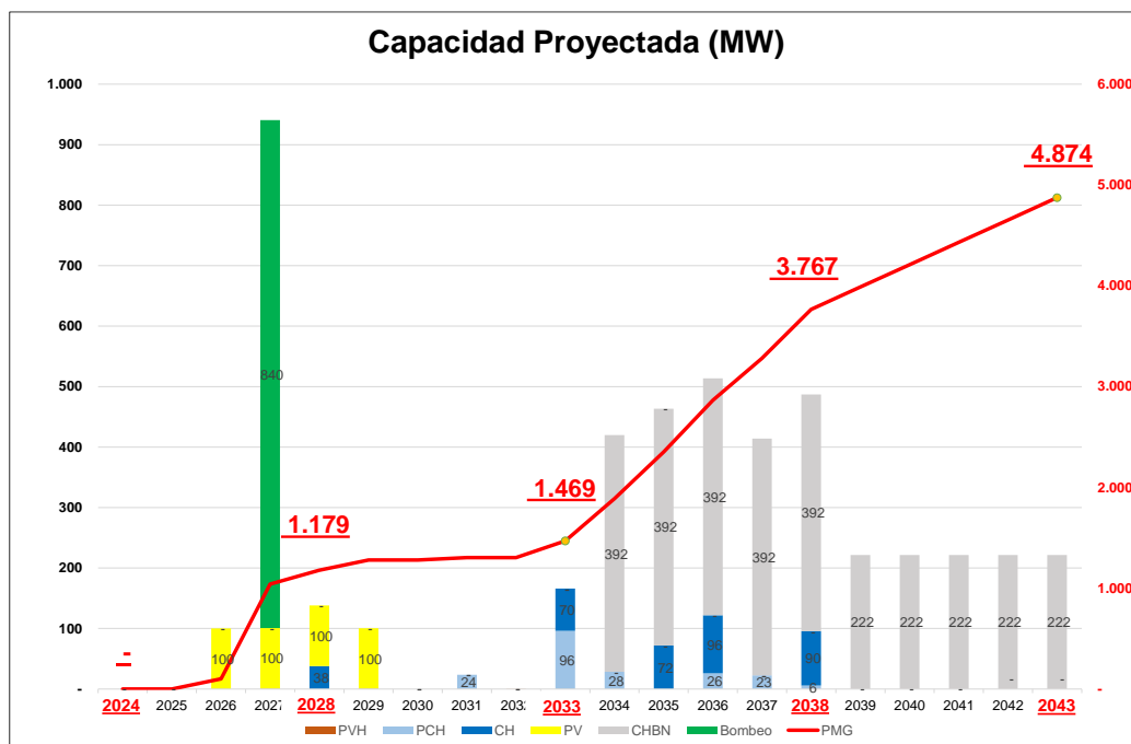
Fig. 4.4 Plan D. Evolución de la Capacidad de Generación 2024-2043.
