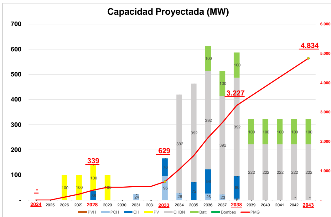
Fig. 4.3 Plan C. Evolución de la Capacidad de Generación 2024-2043.
