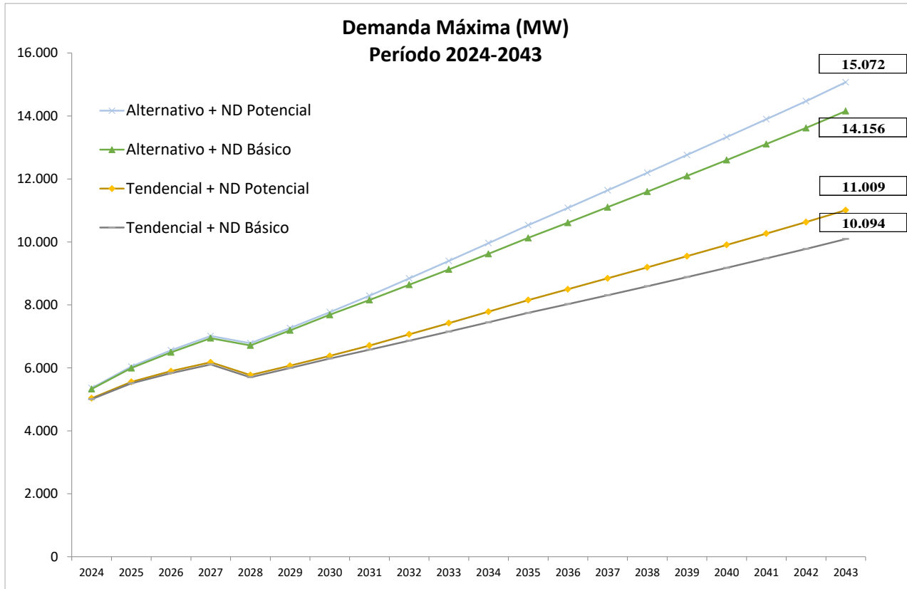
Fig. 2.1 – Proyecciones de la demanda eléctrica 2024-2043.
