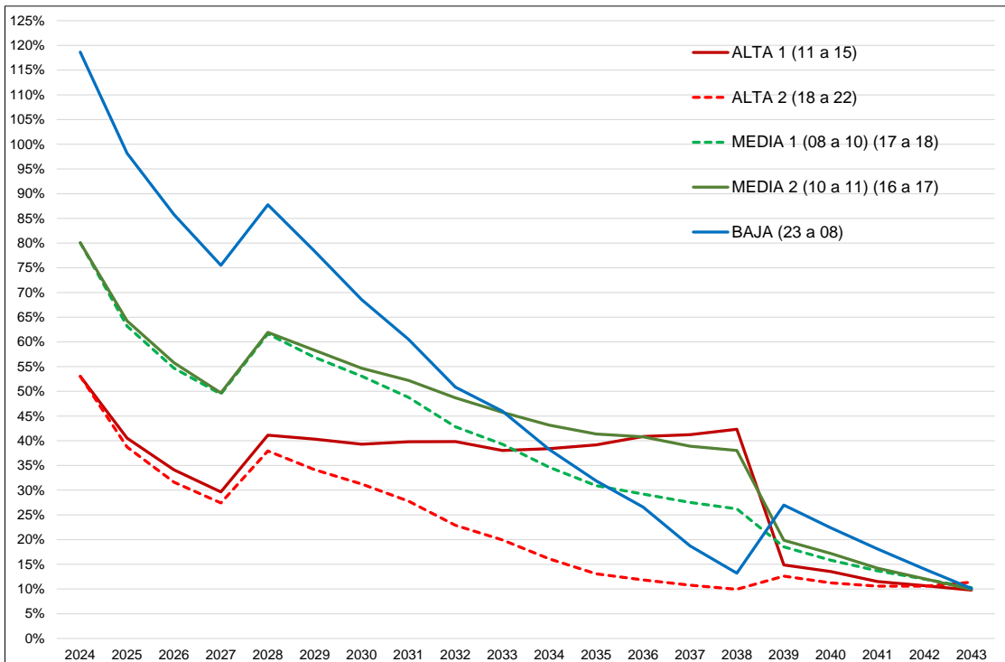
Fig. 4.8 Plan A. Evolución de los Márgenes de Reserva de Potencia (MRP) 2024-2043
