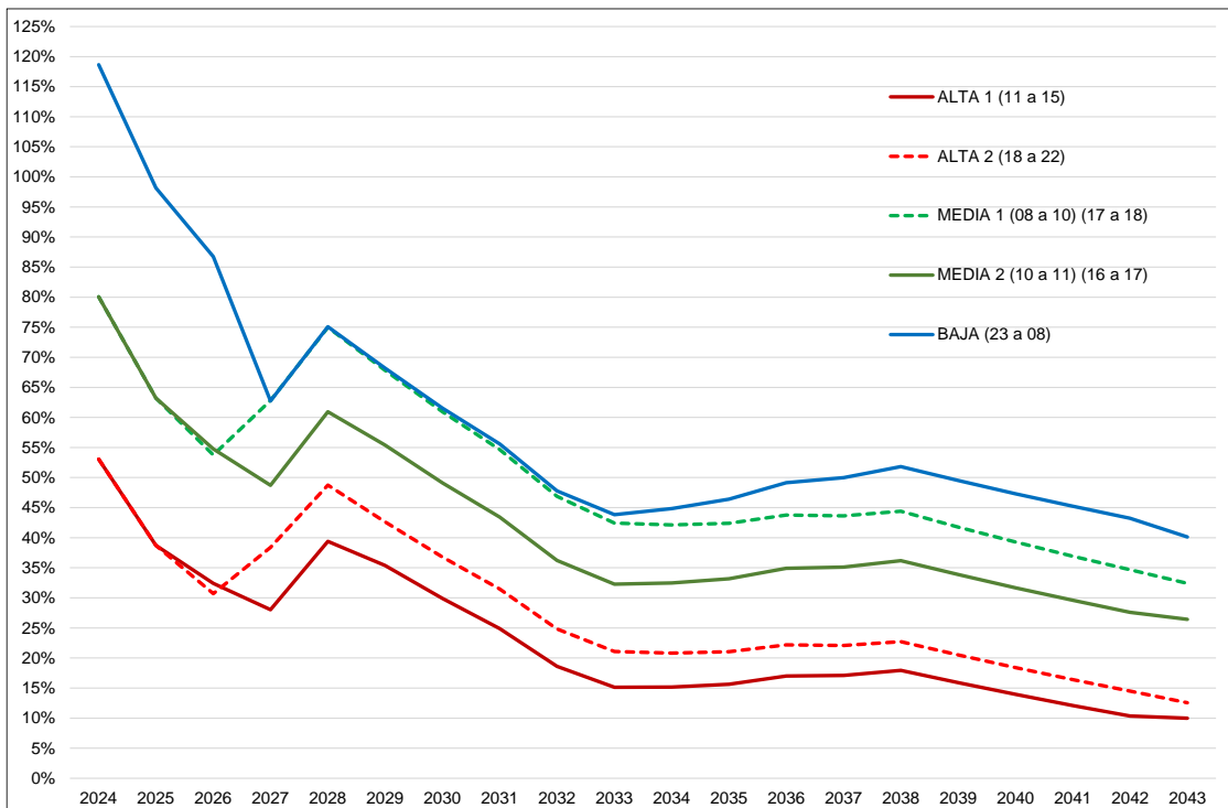
Fig. 4.11 Plan D. Evolución de los Márgenes de Reserva de Potencia (MRP) 2024-2043
