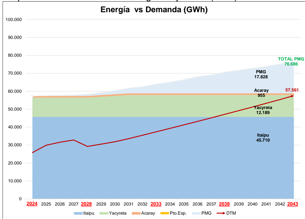
Fig. 4.5 Plan A. Evolución de la Producción de energía esperada 2024-2043.
