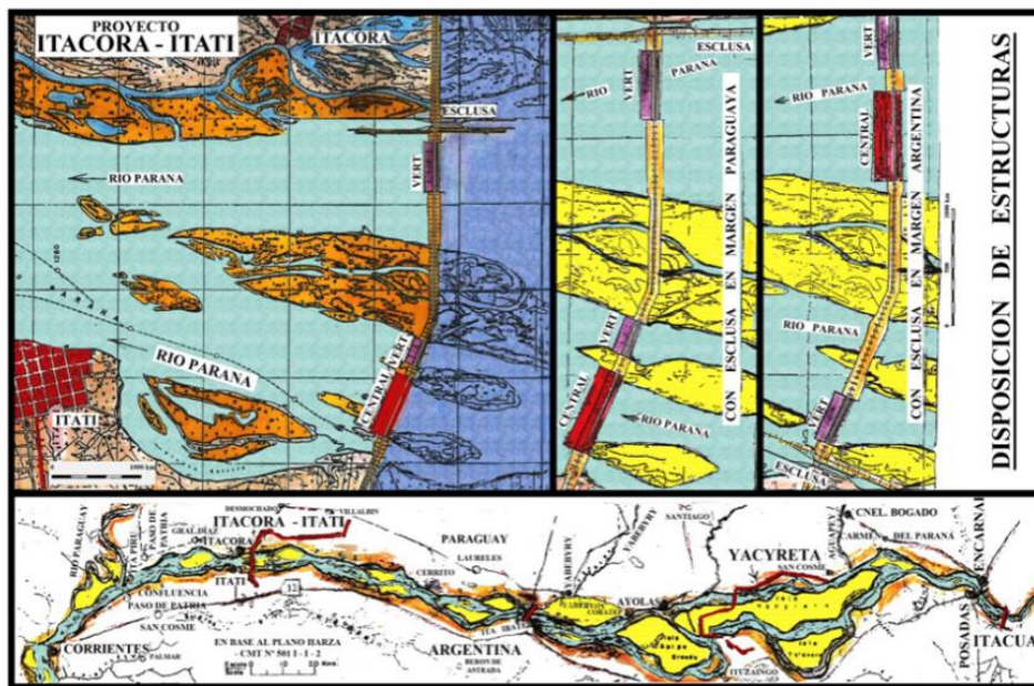
Fig. 3.2 – Ubicación General de la Central Hidroeléctrica de Itacorá-Itatí (CHBN-ItIt)
