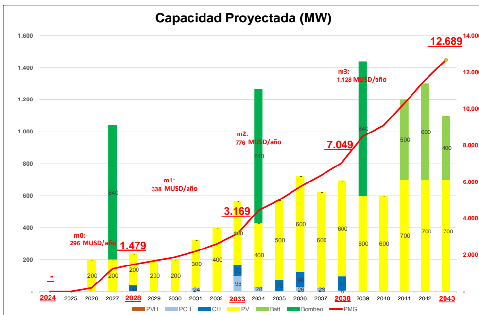
Fig. 4.2 Plan B. Evolución de la Capacidad de Generación 2024-2043.
